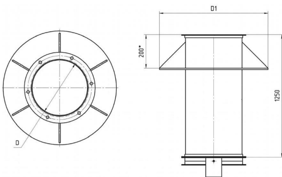
Узел прохода УП-5 с утепленным клапаном под электропривод, без кольца для сбора конденсата
